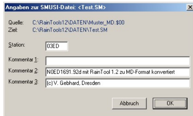
Abb. 7 Konvertierung MD nach SMUSI
