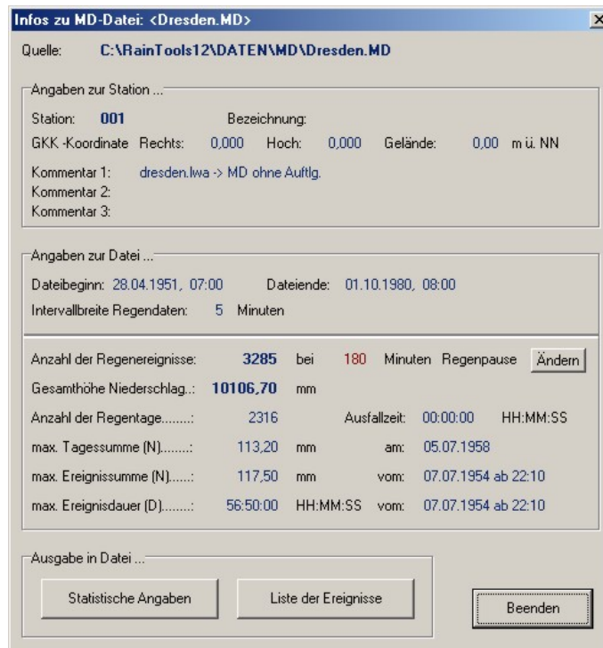
Abb. 16 Ausgabebildschirm Analyse von MD-Dateien
