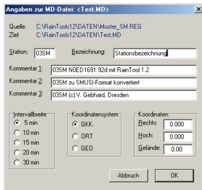
Abb. 8 Konvertierung SMUSI nach MD
